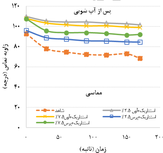
شکل ۳. زاویه تماس قطره آب پیش و پس از آب‌شویی (به مدت ده روز) در سطح شعاعی (الف و ب) و در سطح مماسی (ج و د) چوب بلوط
